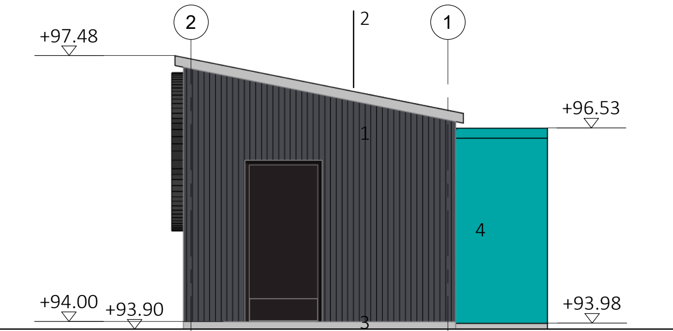
JULKISIVU ITÄÄN
