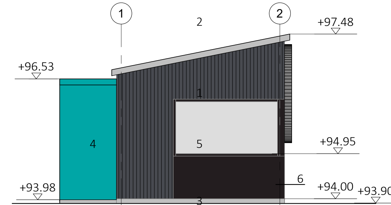
JULKISIVU LÄNTEEN
