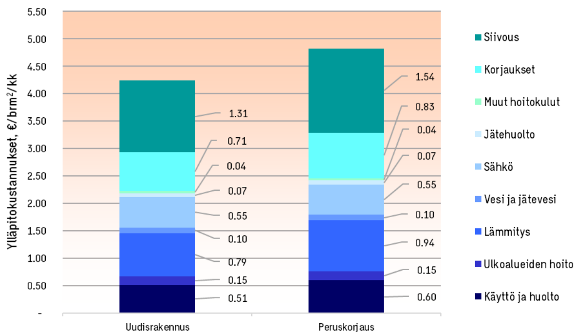
Kuva 6. Elinkaarikustannuslaskennassa käytetyt käyttövaiheen vuotuiset ylläpitokustannukset.
