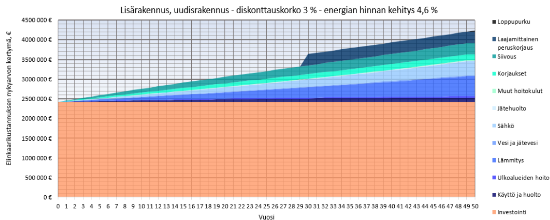
Kuva 20. Elinkaarikustannusten nykyarvon kertyminen 50 vuoden aikana. Lisärakennuksen, uudisrakennus - diskonttauskorko 3% ja energia hinnan kehitys 4,6%.
