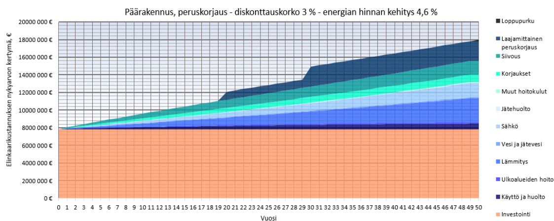
Kuva 13. Elinkaarikustannusten nykyarvon kertyminen 50 vuoden aikana. Päärakennus, peruskorjaus - diskonttauskorko 3% ja energia hinnan kehitys 4,6%.
