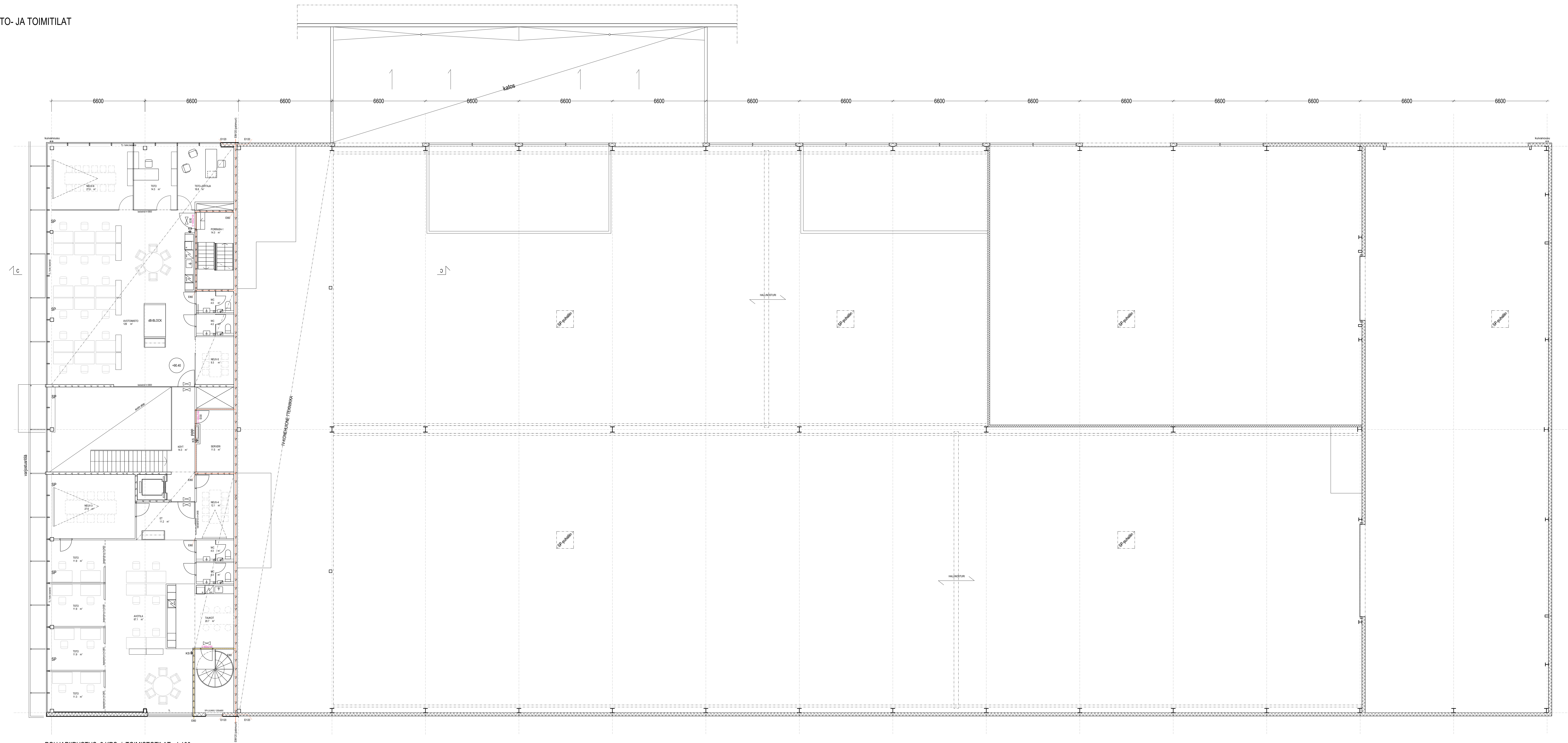
POHJAPIIRUSTUS 2.KRS / TOIMISTOTILAT 1:100
