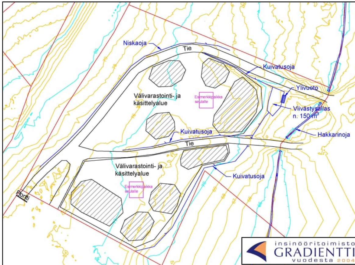
Kuva 9. Vällivarastointialueen asemakuva.
